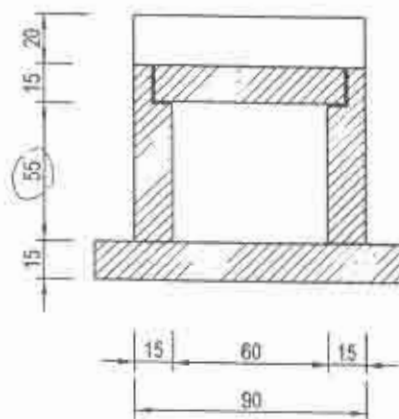
COUPE TRANSVERSALE
