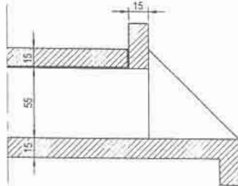
COUPE LONGITUDINALE
