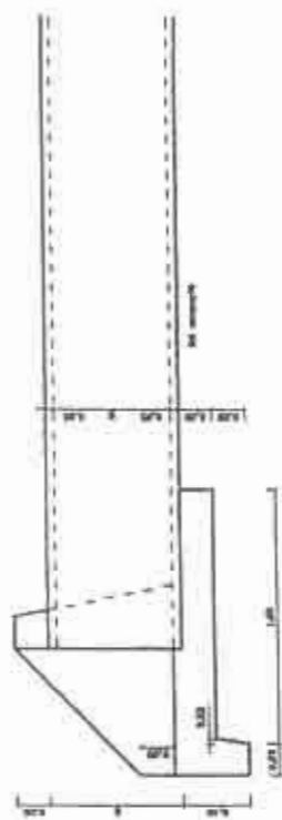
COUPE A-A
